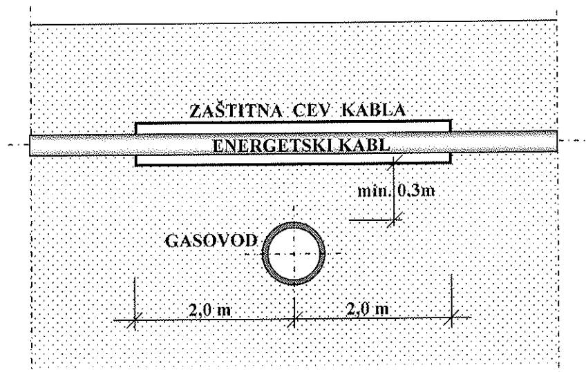
SLUČAJ „B”
