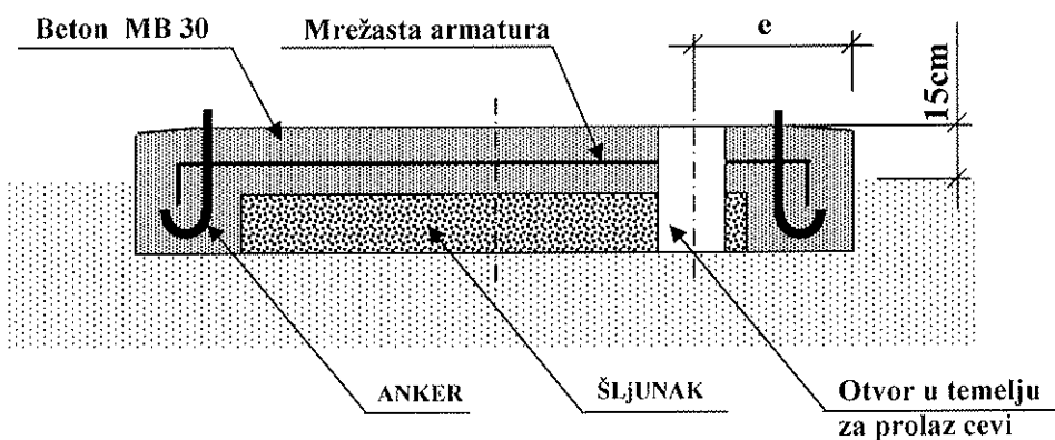
PRESEK B-B
