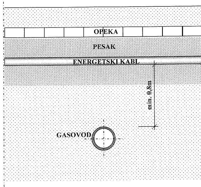
SLUČAJ „A”
