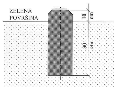
DETALJ OZNAKE GASOVODA U NASELJENOM MESTU U TROTOARU I NA ZELENOJ POVRŠINI
