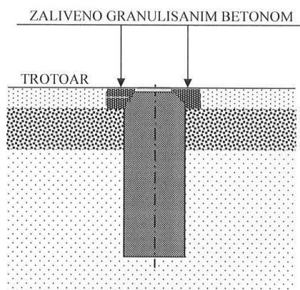
DETALJ OZNAKE GASOVODA U NASELJENOM MESTU U TROTOARU I NA ZELENOJ POVRŠINI
